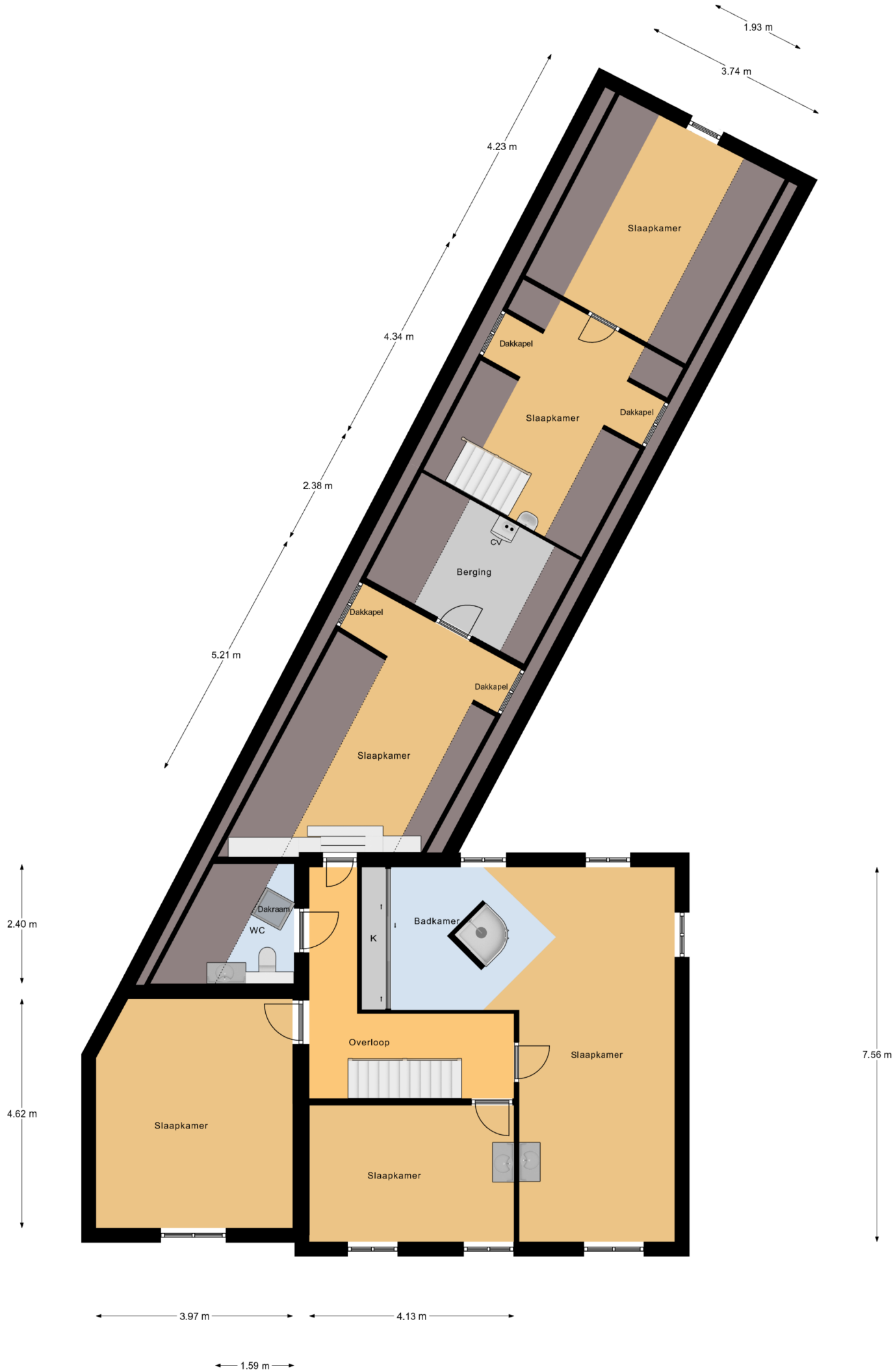
1e Verdieping
